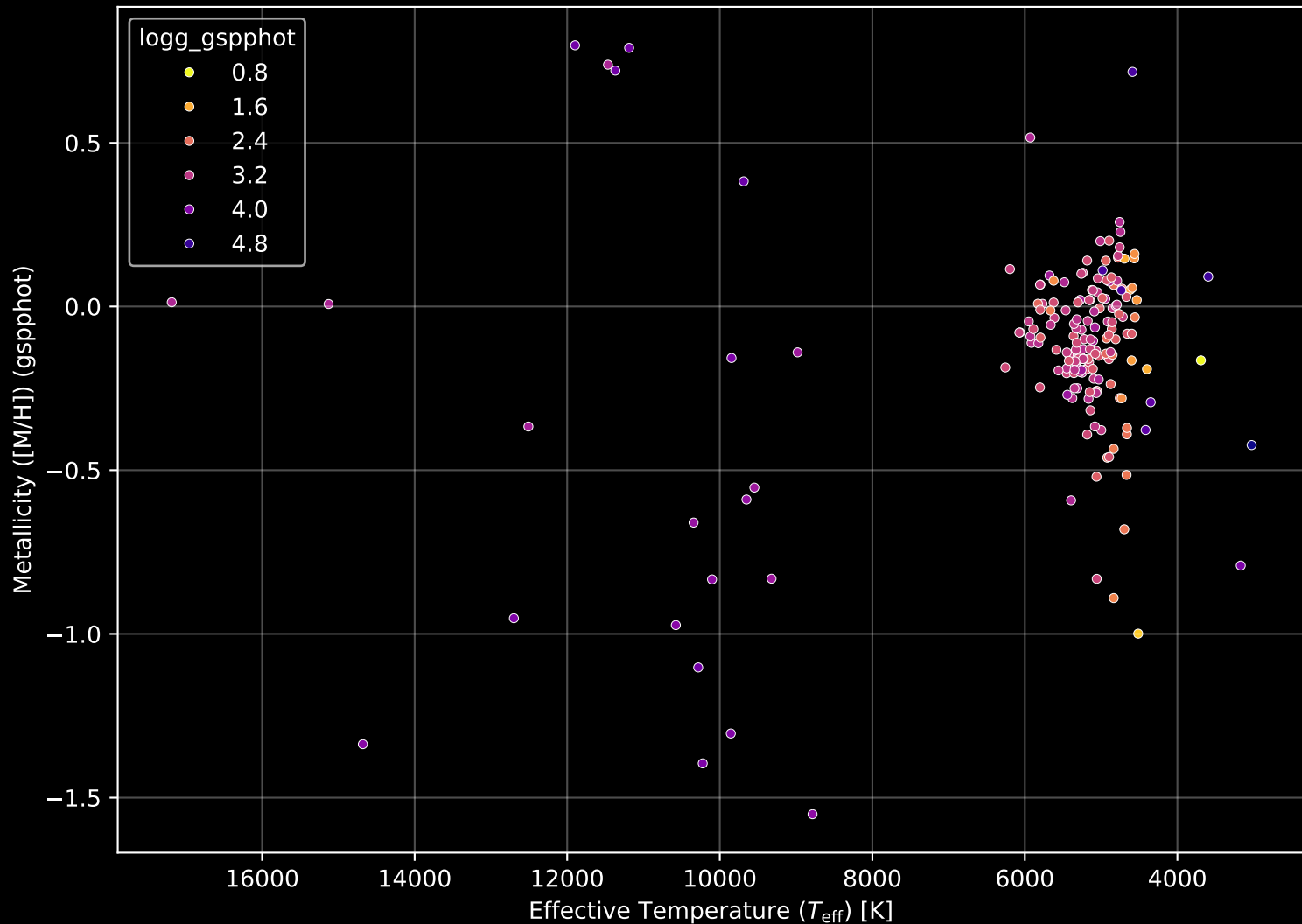
APOGEE DR17 Field: [184+04] Stellar Population Parameters (n= 186)
